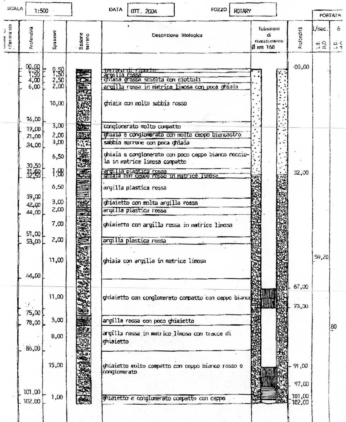
Fig. 5.5 – Stratigrafia pozzo Cooperativa Acquisport
