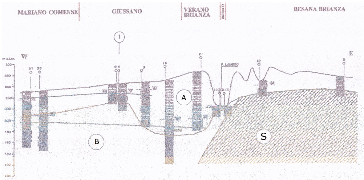
Fig. 5.3 – Sezioni idrogeologiche trasversali 2 e 3 - scala lunghezza 1:3500 circa (tratto da Ghezzi 2007, modificato)
