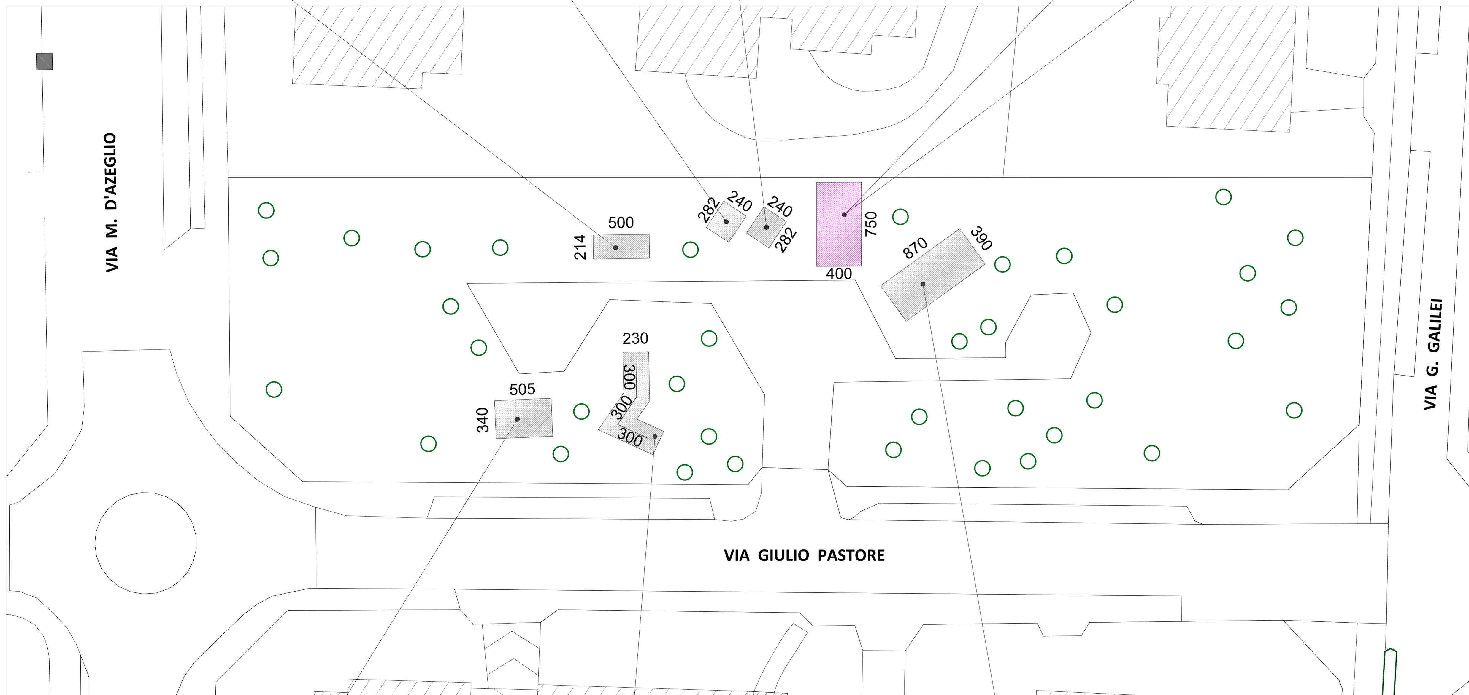
PLANIMETRIA GENERALE OPERE DI URBANIZZAZIONE SECONDARIA PRESSO IL PARCO GIOCHI PUBBLICO DI VIA GIULIO PASTORE SCALA 1:200
